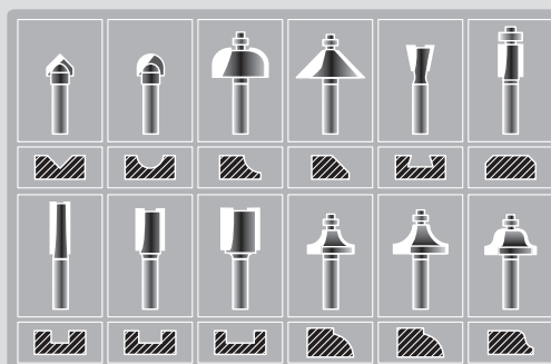
Abb. 1, Profilform an Abhängigkeit vom eingesetzten Profilfräser
