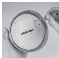
Odšroubujte kryt baterií
