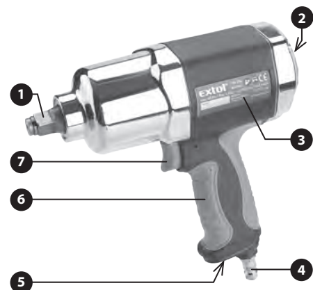
Obr. 3, popis modelu uťahovávka WI 680
