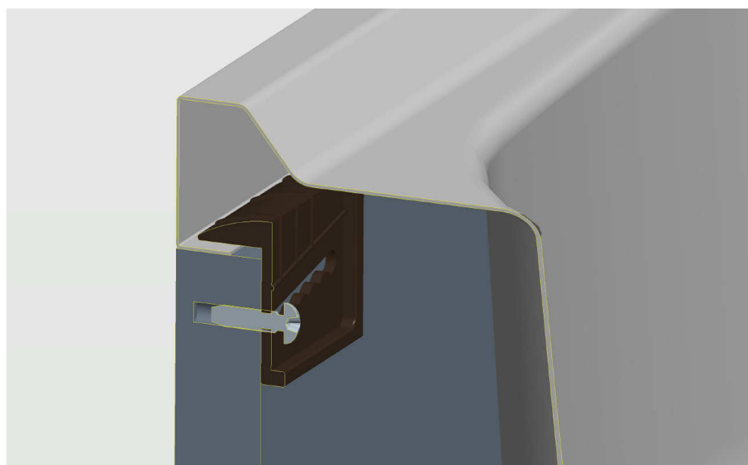
4. Vstavljanje pritrdilca skozi vijak
