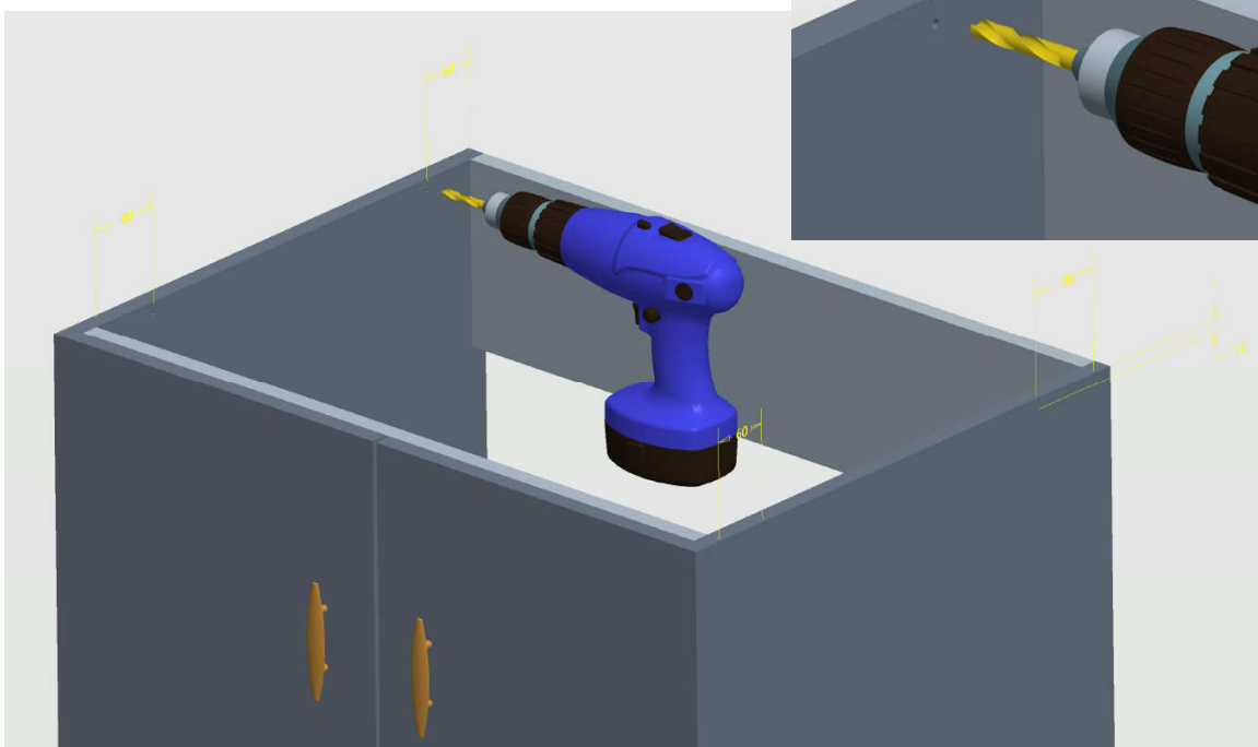
1. Vrtanje lukenj v omarico
