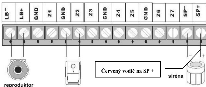
příklad zapojení jednoho z detektorů
